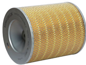
OEM NO. : 4L-9852 AUTOCOM NO: AIL-4L-9852 CAT (5505) SIZE(OD*ID*H) : 265*153*317mm
