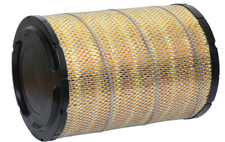
OEM NO. : 131-8822 AUTOCOM NO: AIL-131-8822 CAT (8508) SIZE(OD*ID*H) : 237*132*343mm
