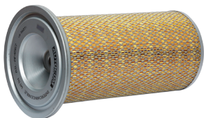
OEM NO. : 4I-7575 AUTOCOM NO : AIL-4567 CAT (5627) SIZE(OD1*OD2*ID*H) : 236*186*118*393mm
